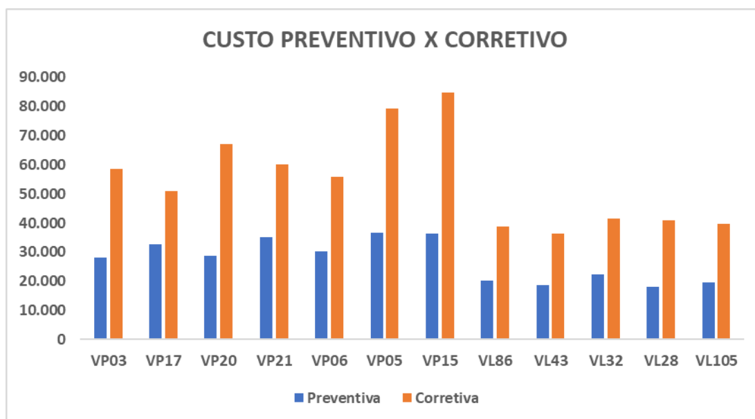
GRÁFICO 6 – CUSTO PREVENTIVO X CORRETIVO DA FROTA.
