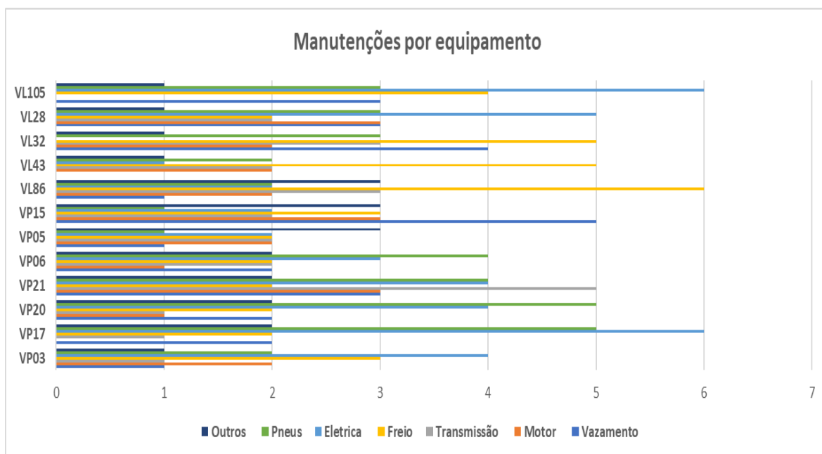
GRÁFICO 2 – TIPOS DE MANUTENÇÕES POR SISTEMAS.
