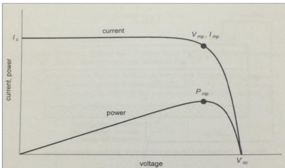
Figura 3 - Curva típica do comportamento da célula
