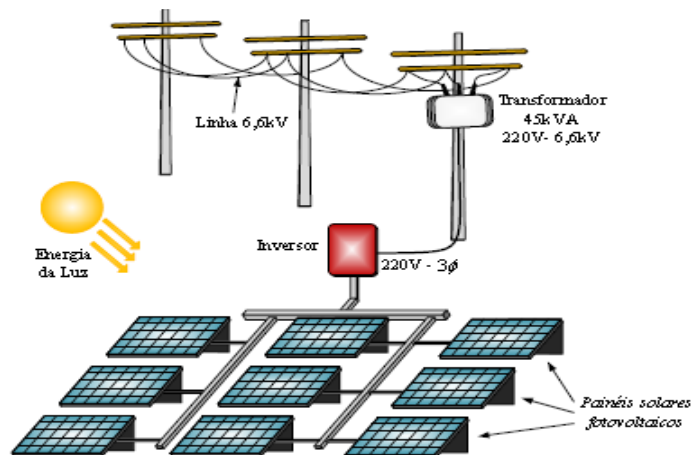
Figura 9 – Diagrama esquemático do Laboratório Solar Fotovoltaico da UFJF
