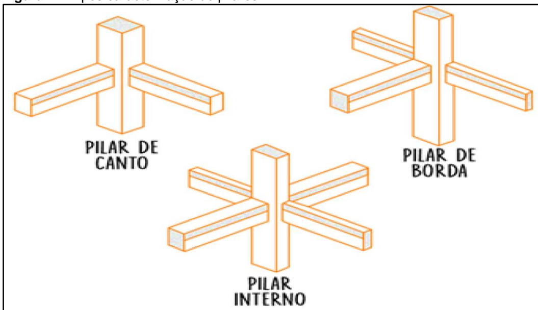
Figura 7 – Tipos caracterização de pilares
