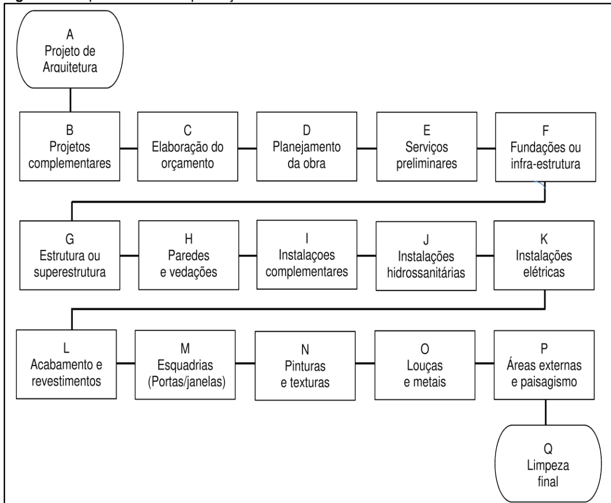
Figura 1 - Etapas básicas à implantação de uma obra civil
