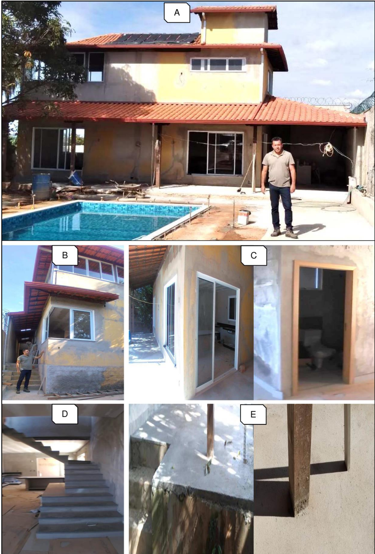
Figura 17 - Ilustração/resultado visual das recomendações que foram implementadas
