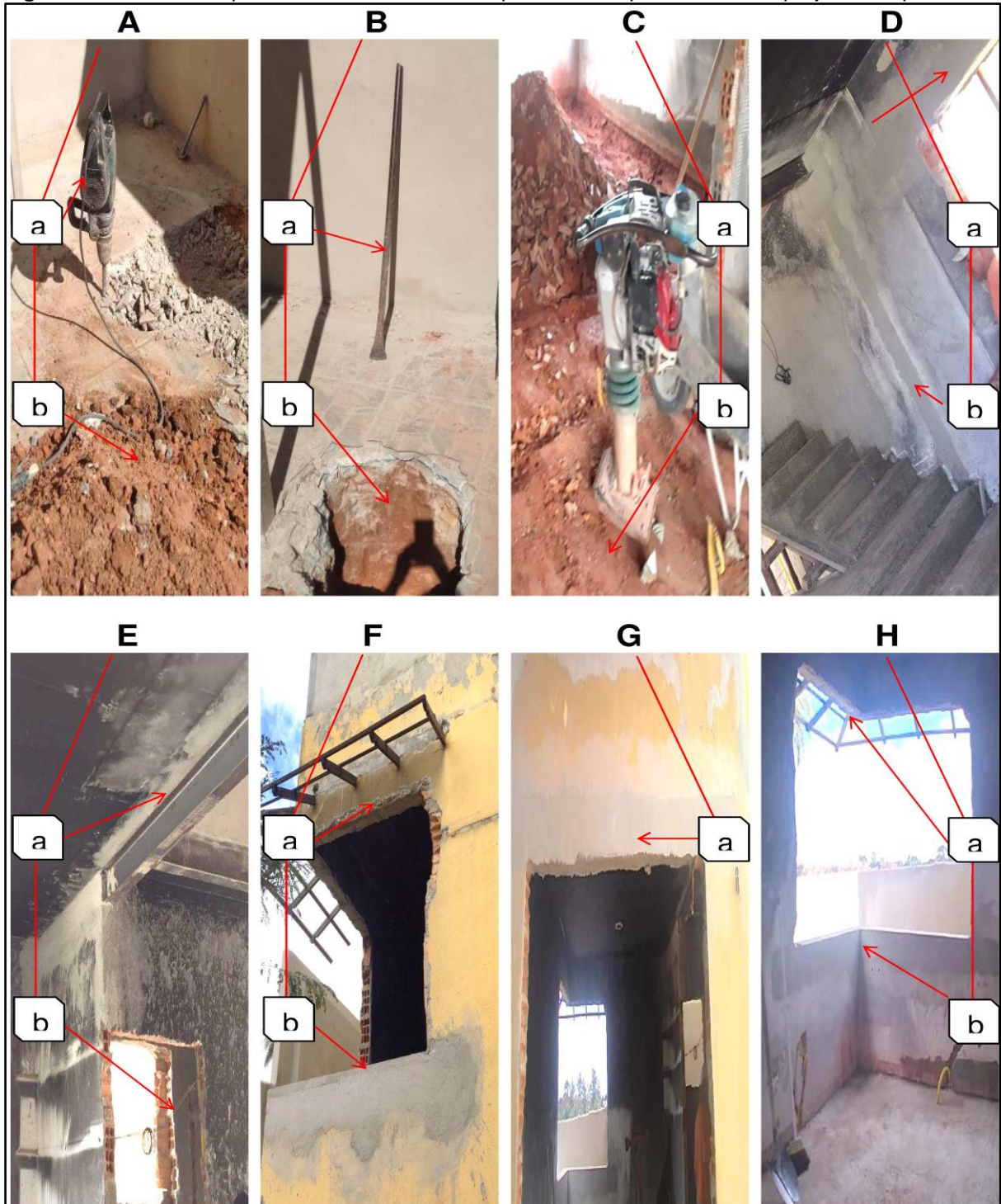
Figura 16 - Acompanhamento sobre o que foi requisitado no projeto arquitetônico
