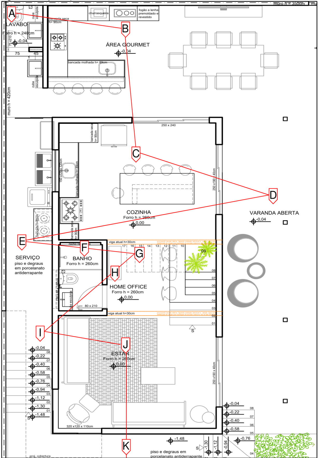
Figura 14 - Projeto arquitetônico – Pavimentos 1 e 2
